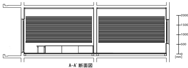
A-A' 断面図
