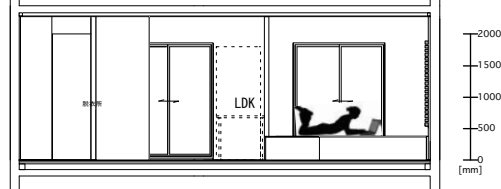
B-B' 断面図
